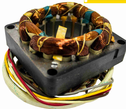
RLB-0274 REF A 7.75 PZA |BOBINA VENTILADOR MET.CUADRADA 25MM REF B=11.79 REF C=12.41
