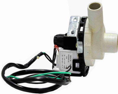
RLB-0250 REF A 18.72 PZA |BOMBA 35w P/DESAGUE LAVADOR DAKA R REF B=28.5 REF C=30
