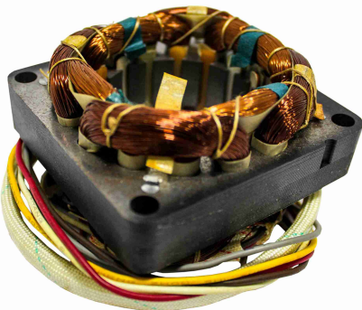
RLB-0272 REF A 7.75 PZA |BOBINA VENTILADOR MET.CUADRADA 18MM REF B=11.79 REF C=12.41
