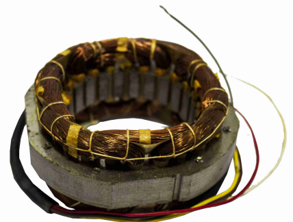
RLB-0280 REF A 2.78 PZA |BOBINA VENTILADOR MET.REDONDA 18MM REF B=4.23 REF C=4.45
